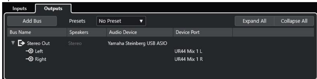
Outputs tab
